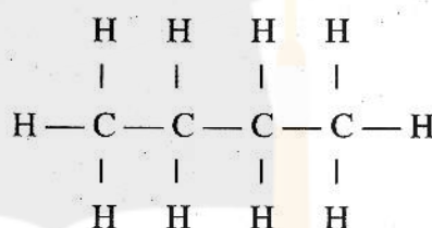
Butane
