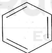
(Benzene)
